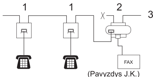
2 pav.: Rekomenduojamas plėtinių lizdų sujungimas
