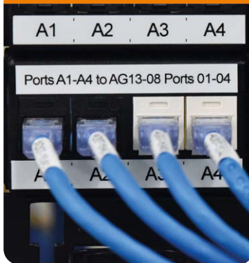
Liitäntöjen merkitseminen
